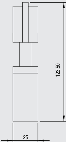
Неправильная Установка / Worong Assembly
