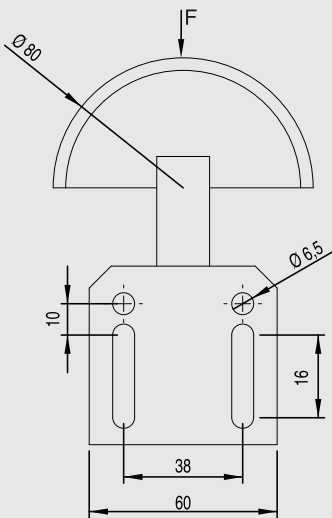
Неправильная Установка / Worong Assembly
